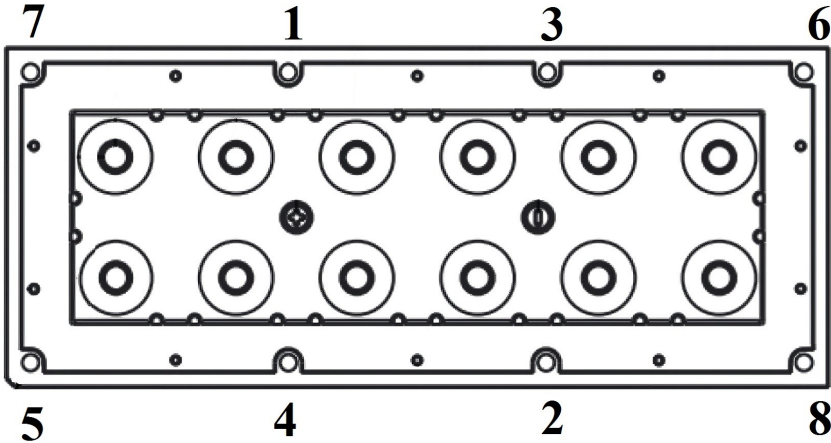
Чертёж линзы
