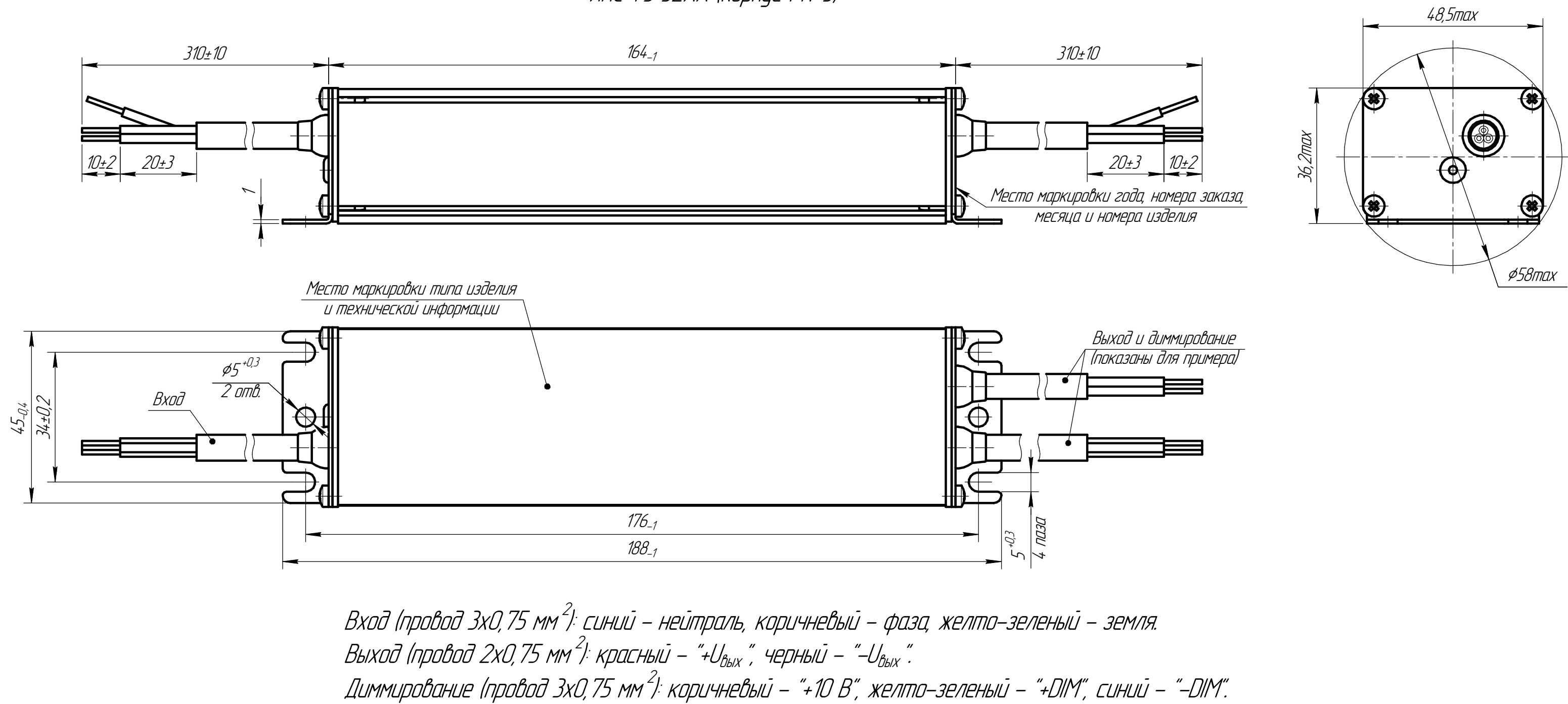
ИПС ТУ 52XX (корпус PN-3)
