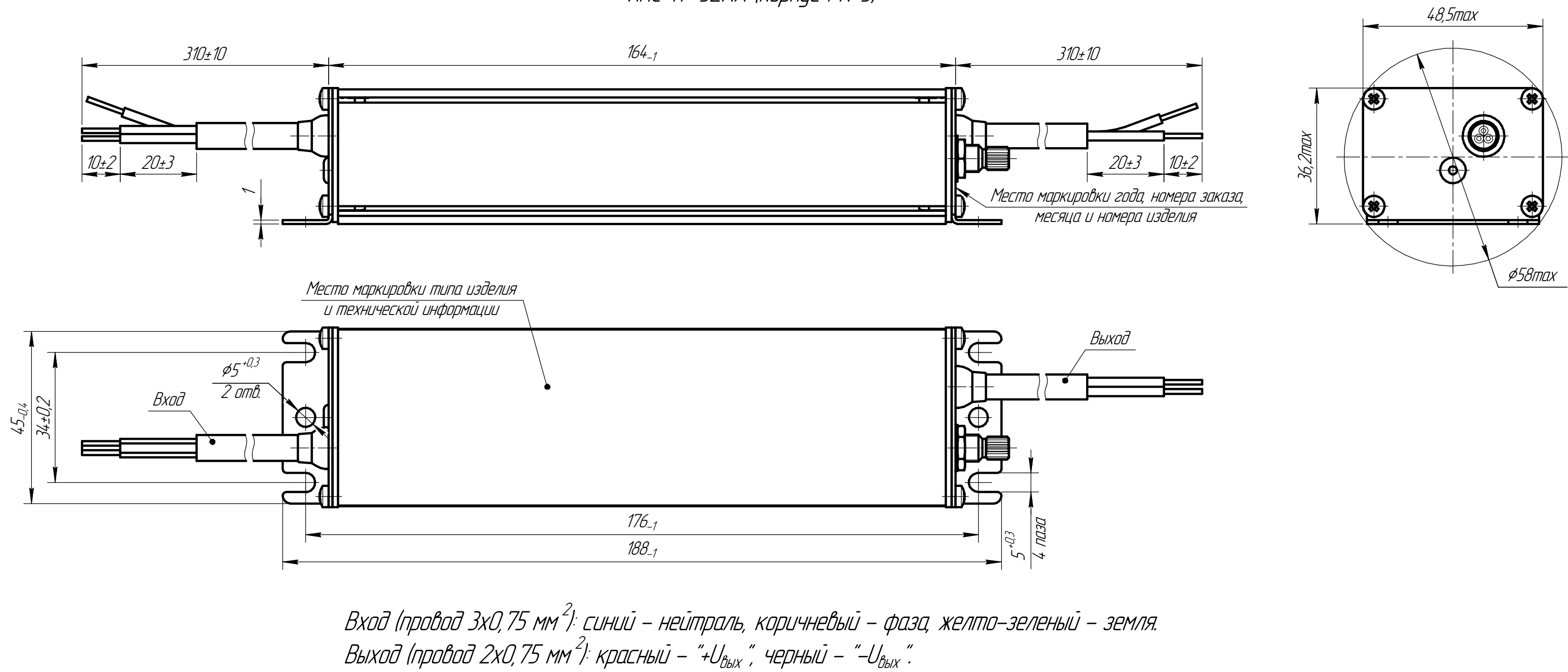
ИПС ТР 52XX (корпус PN-3)
