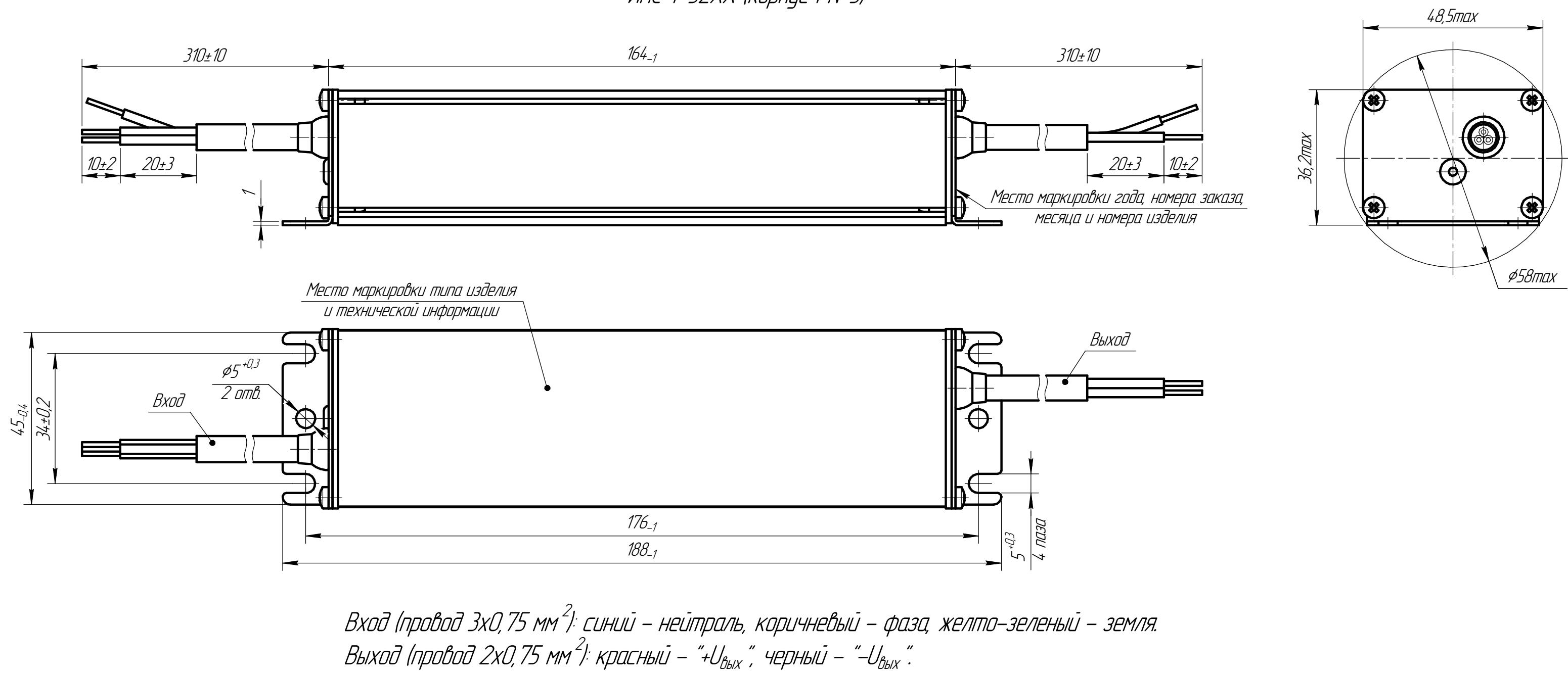
ИПС Т 52XX (корпус PN-3)
