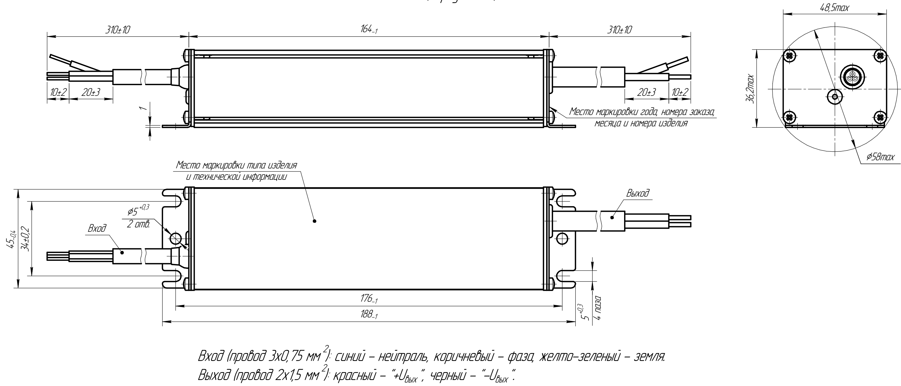
ИПС Н 52XX (корпус PN-3)
