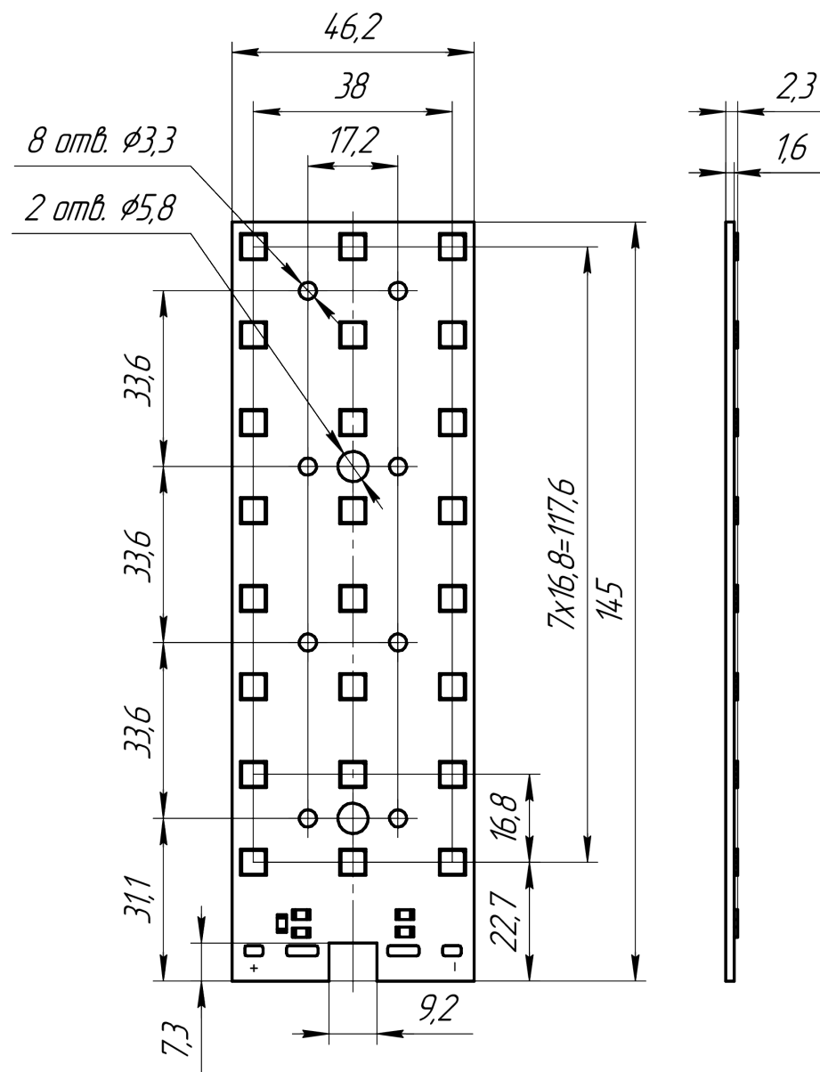
ПРИЛОЖЕНИЕ А Чертеж светодиодного модуля под пайку
