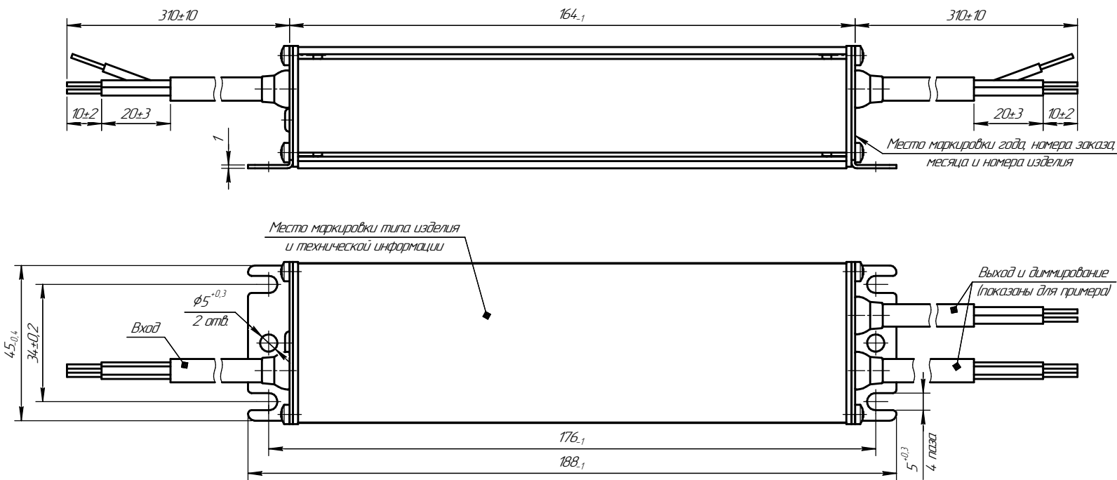
ИПС ТУ 52XX (корпус PN-3)
