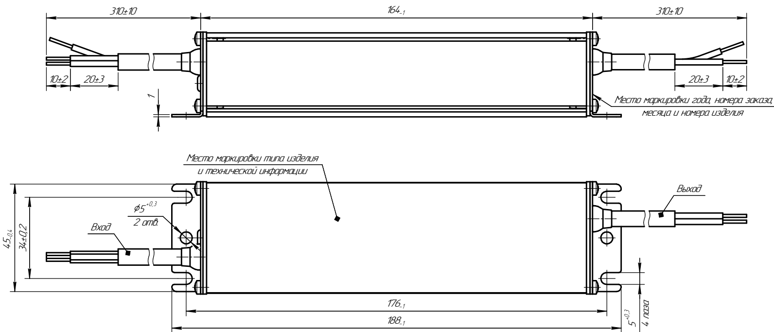
ИПС Т 52XX (корпус PN-3)
