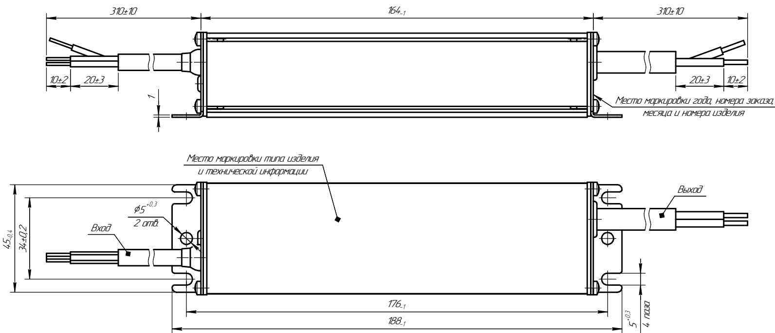
ИПС Н 52XX (корпус PN-3)
