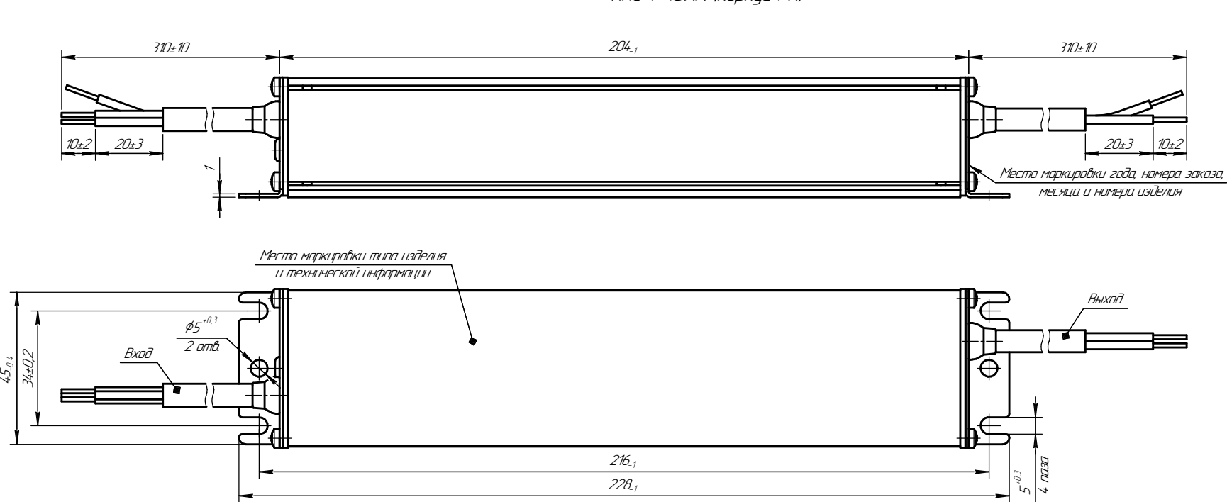
ИПС Т 43XX (корпус РN)
