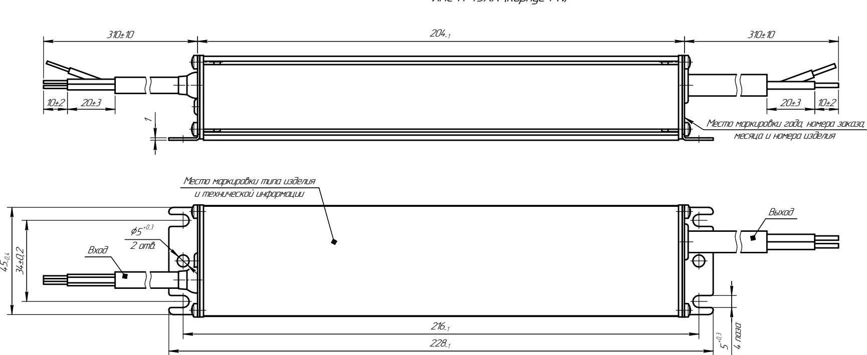
ИПС Н 43XX (корпус РN)
