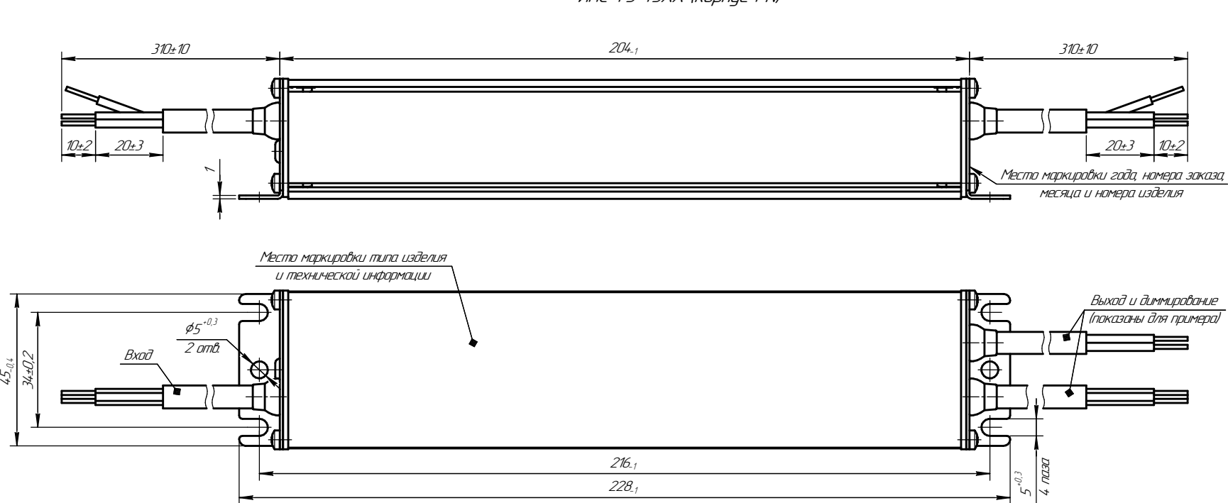
ИПС ТУ 43XX (корпус РN)
