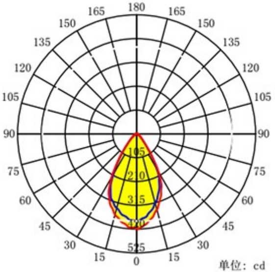
ДИАГРАММА РАСПРЕДЕЛЕНИЯ СИЛЫ СВЕТА
