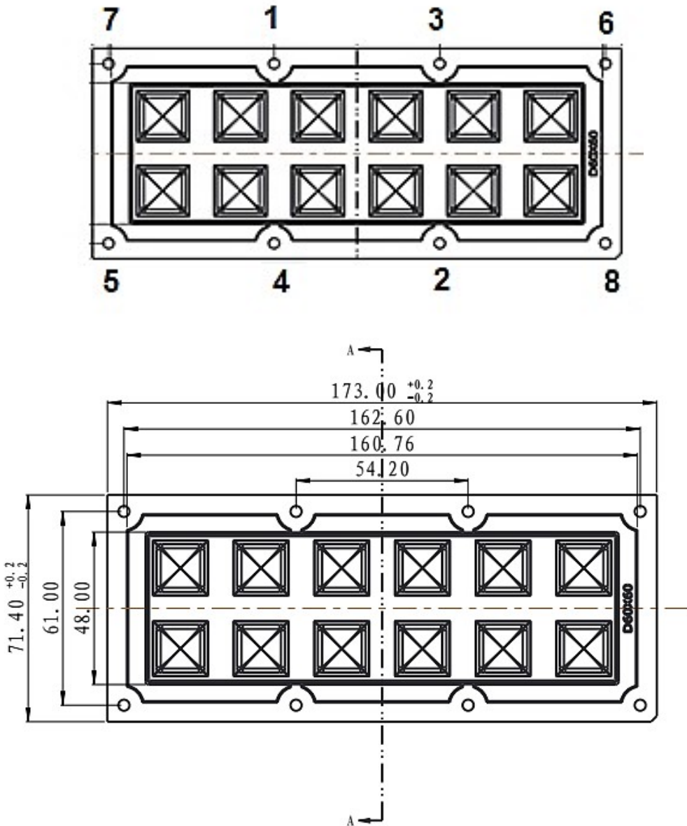
Чертёж линзы
