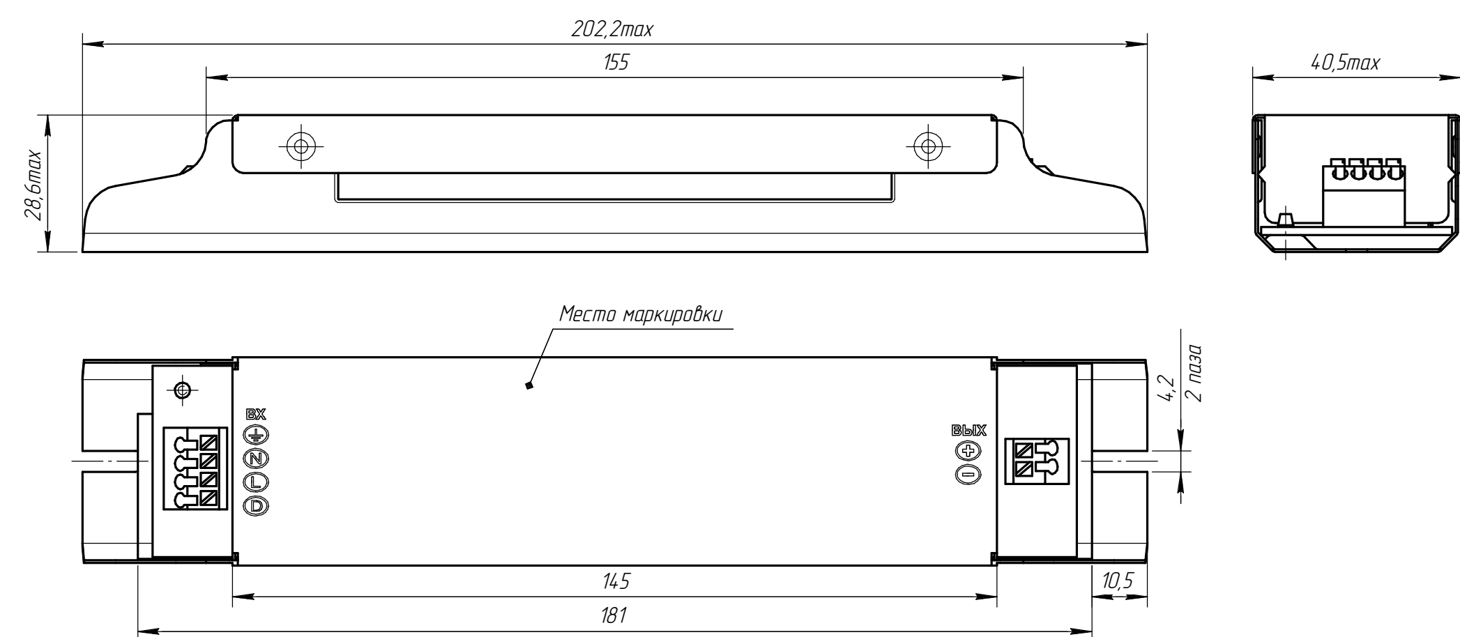
ИПС ТИ 0104 (корпус А)
