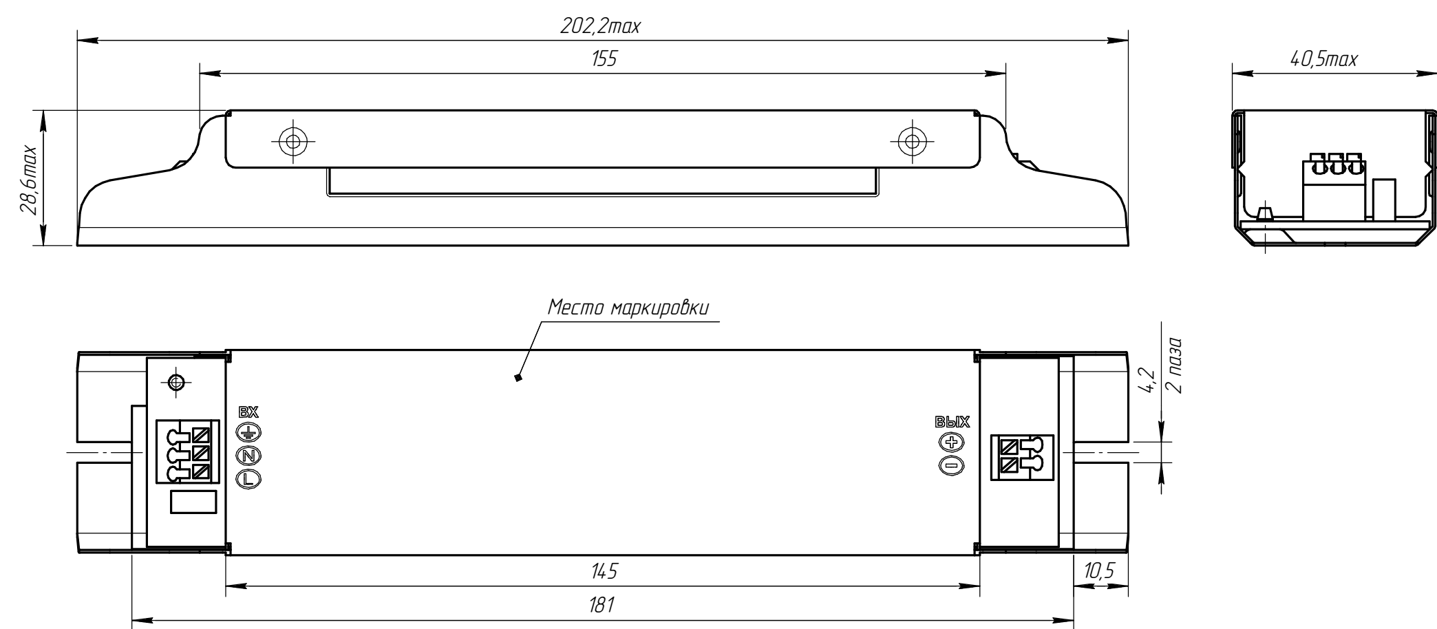
ИПС Т 0100, 0105 и Т 0ФИС 0110, 0111 (корпус А)
