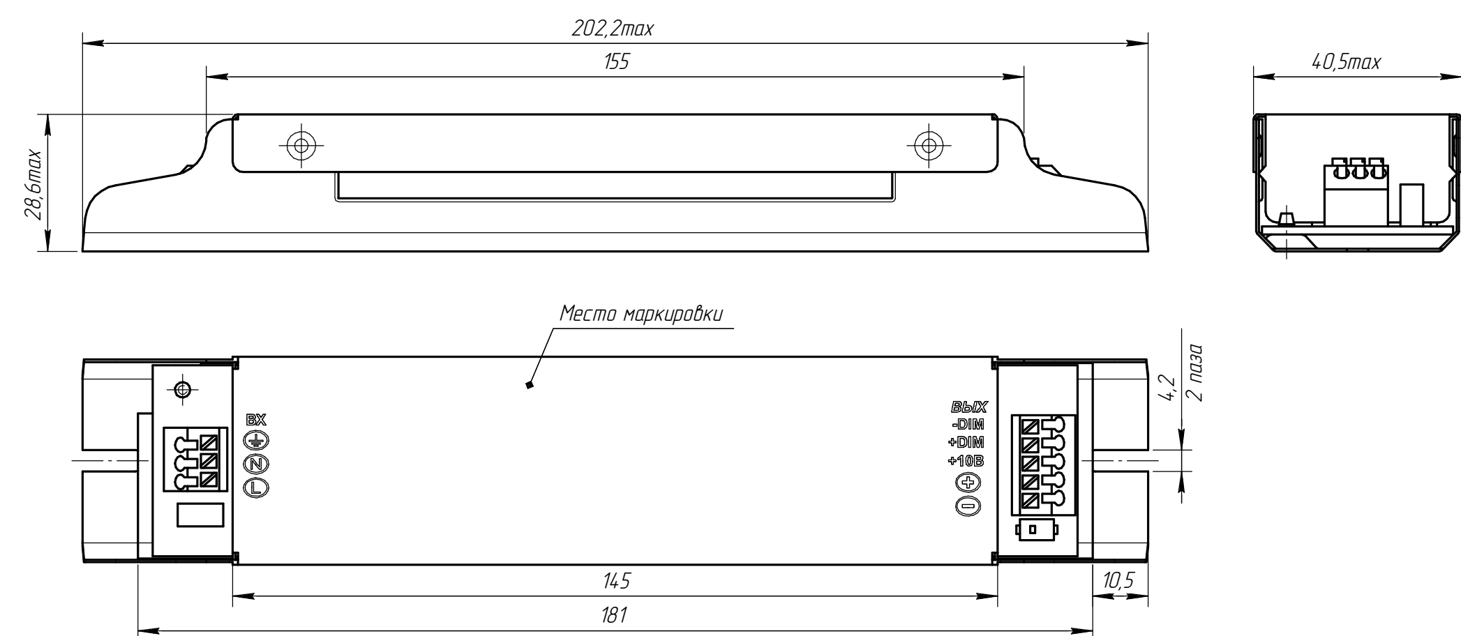
ИПС 60 Вт ТУ 0102 (корпус А)
