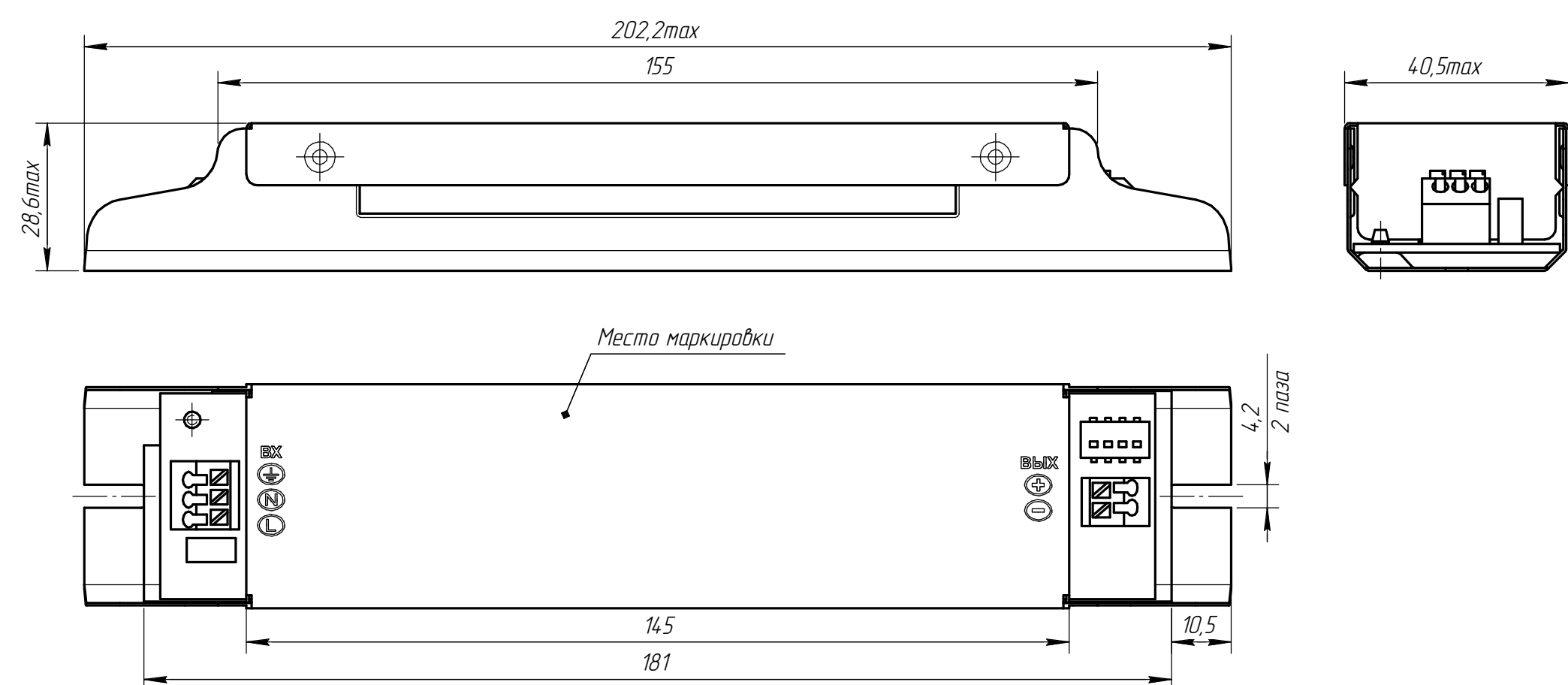
ИПС 40-50 Вт ТД 0100, 0105 (корпус А)
