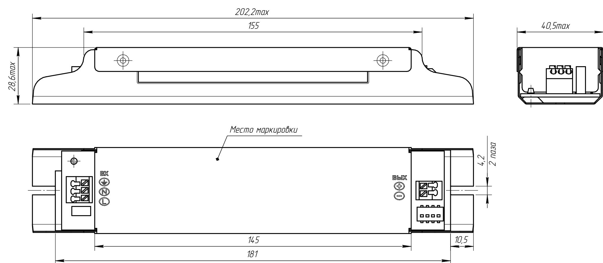
ИПС 60 Вт ТД 0100, 0105 (корпус А)
