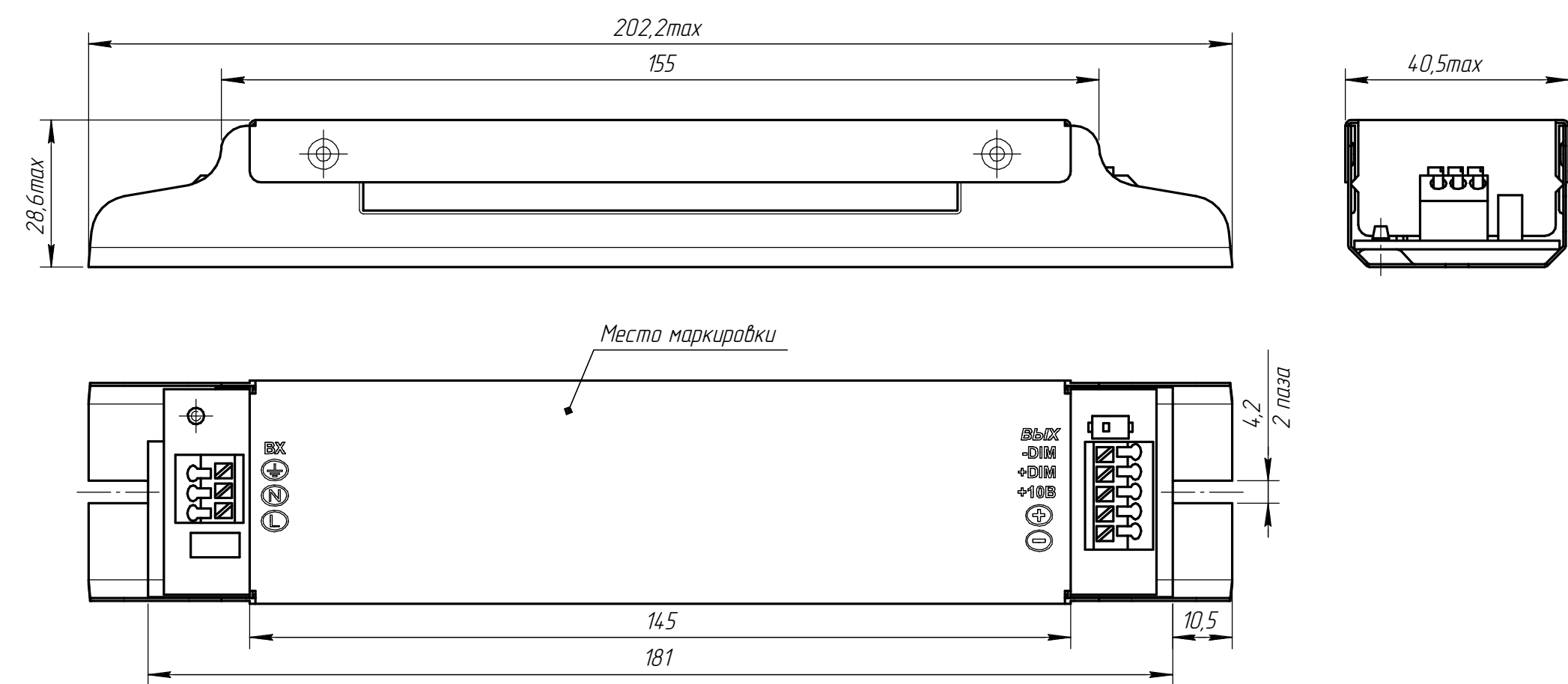
ИПС 50 Вт ТУ 0102 (корпус А)
