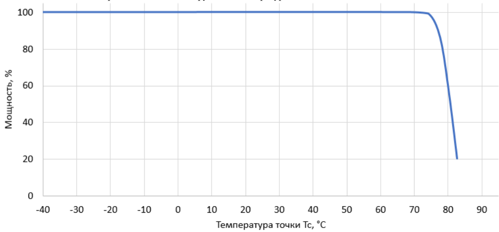
Зависимость мощности при максимальной нагрузке от температуры точки Тс.
