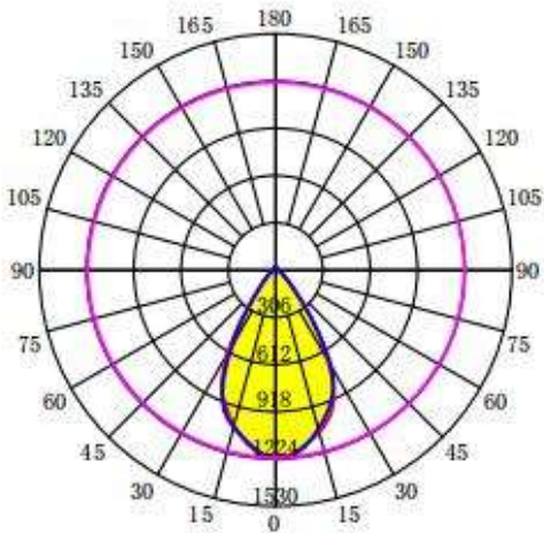
配光曲线
