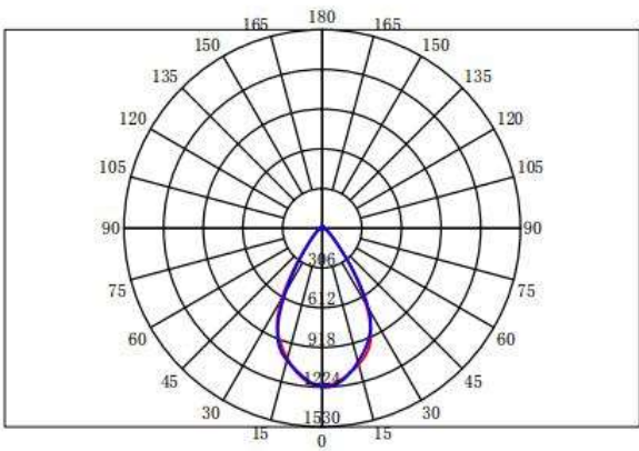
配光曲线
