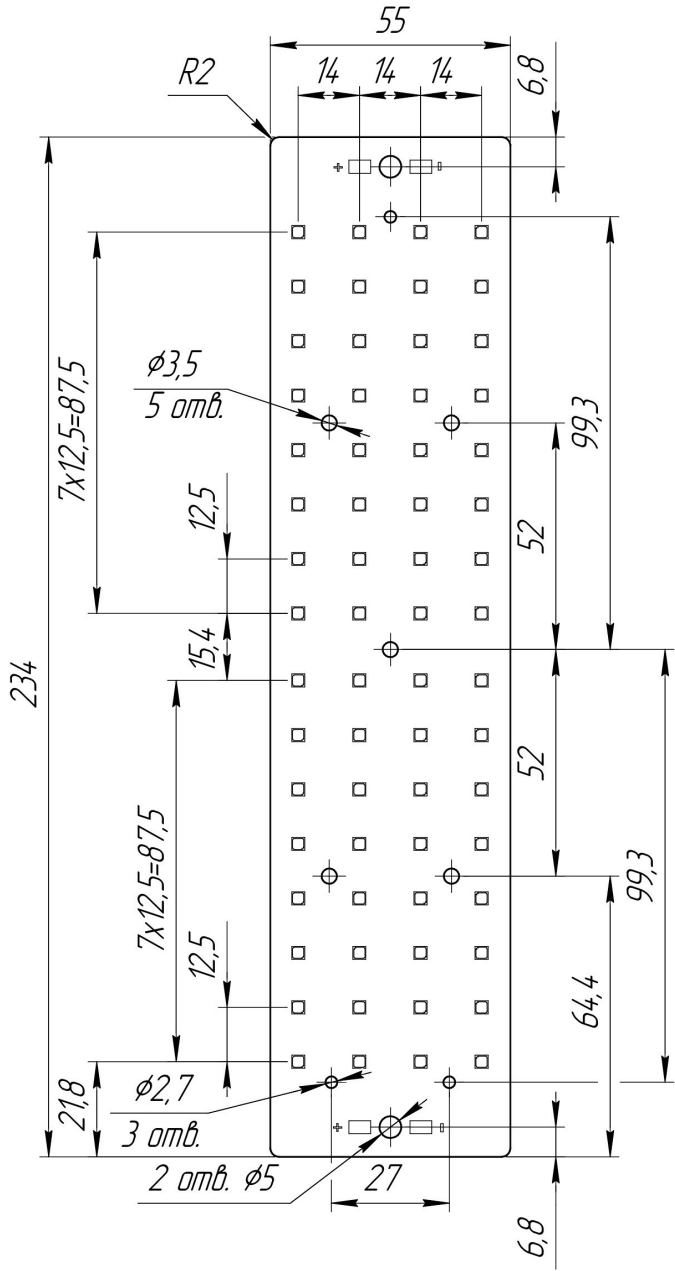
ПРИЛОЖЕНИЕ А Чертеж светодиодного модуля
