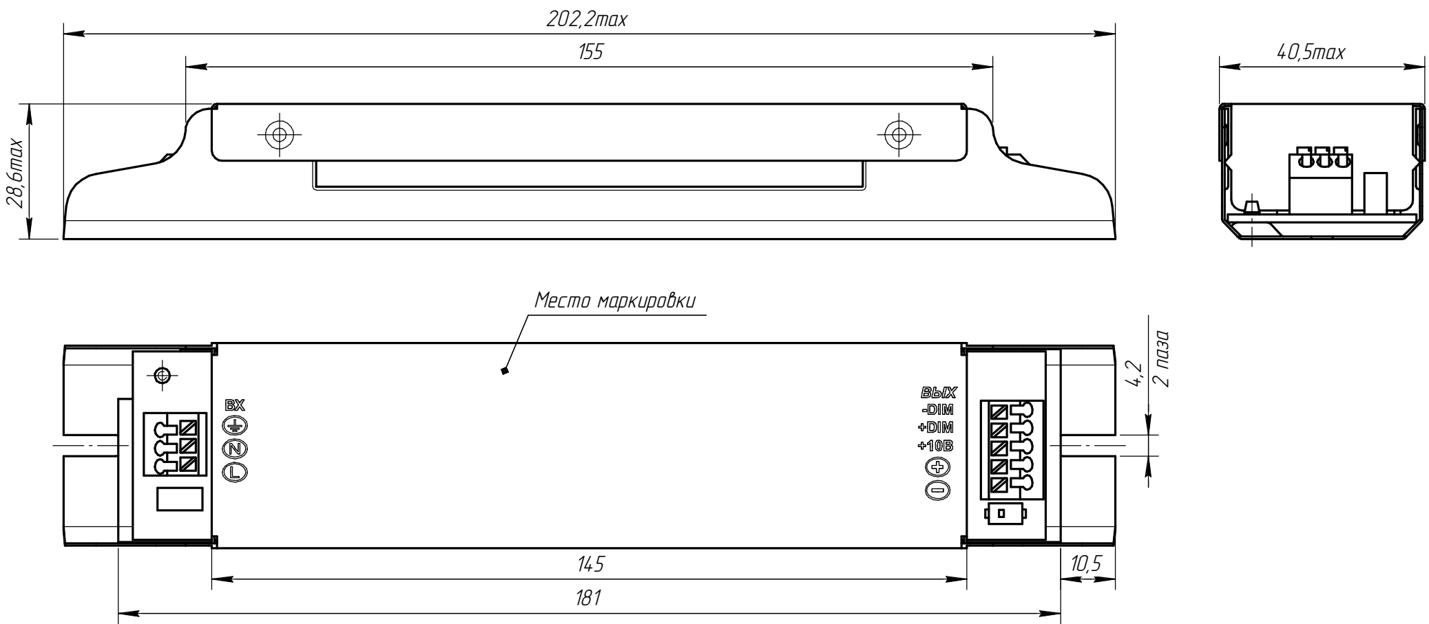
ИПС 60 Вт ТУ 0102 (корпус А)
