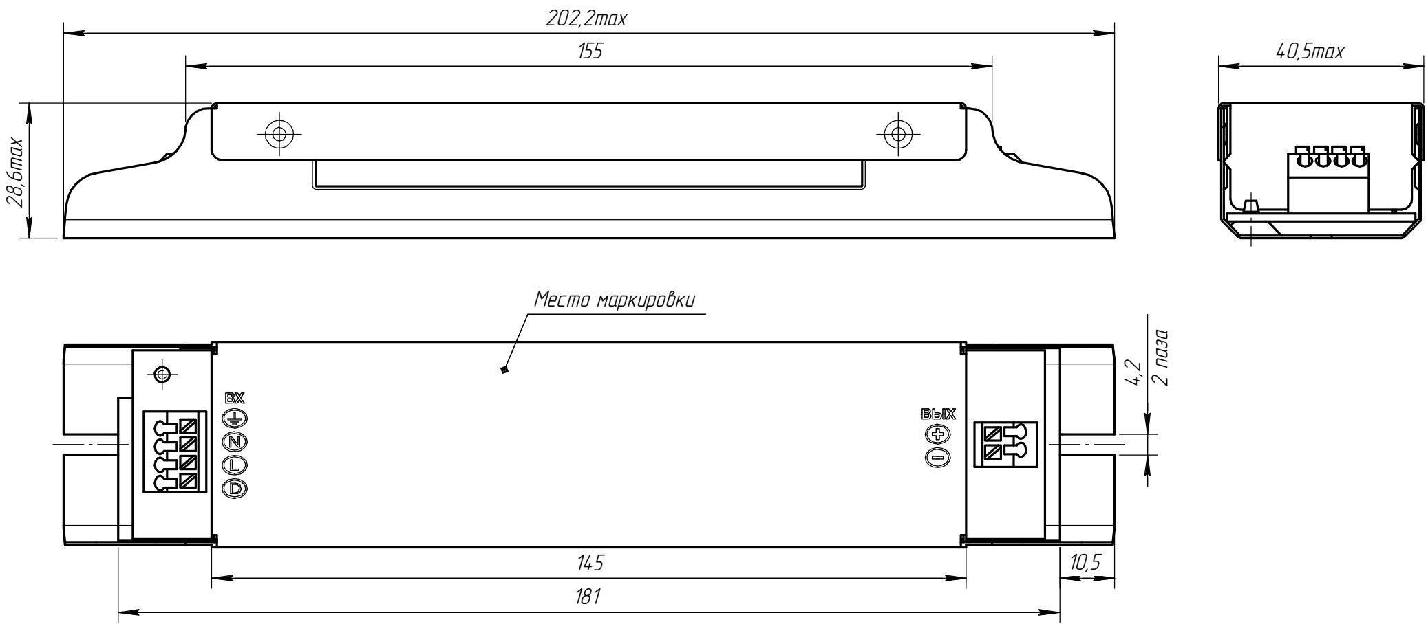
ИПС ТИ 0104 (корпус А)
