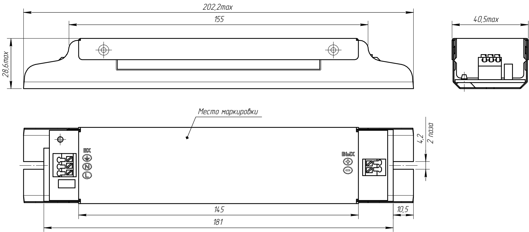
ИПС Т 0100, 0105 и Т 0ФИС 0110, 0111 (корпус А)
