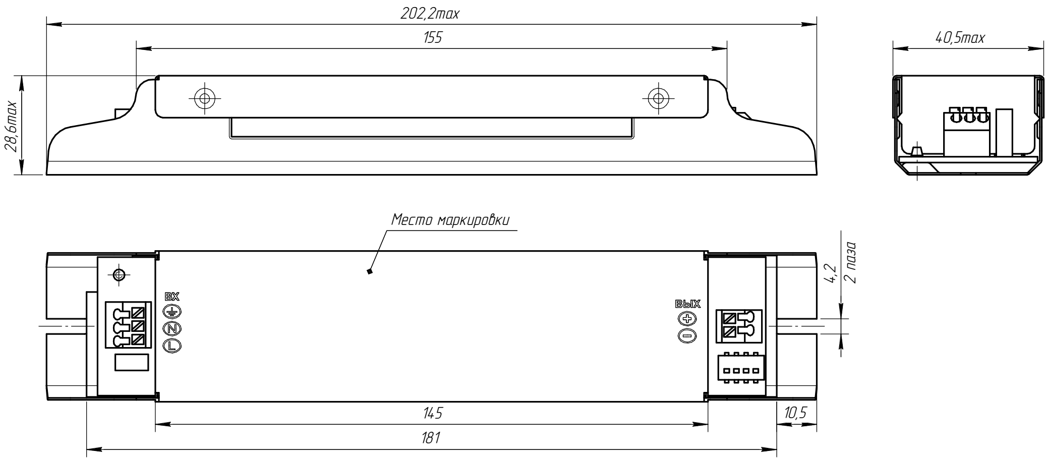
ИПС 60 Вт ТД 0100, 0105 (корпус А)
