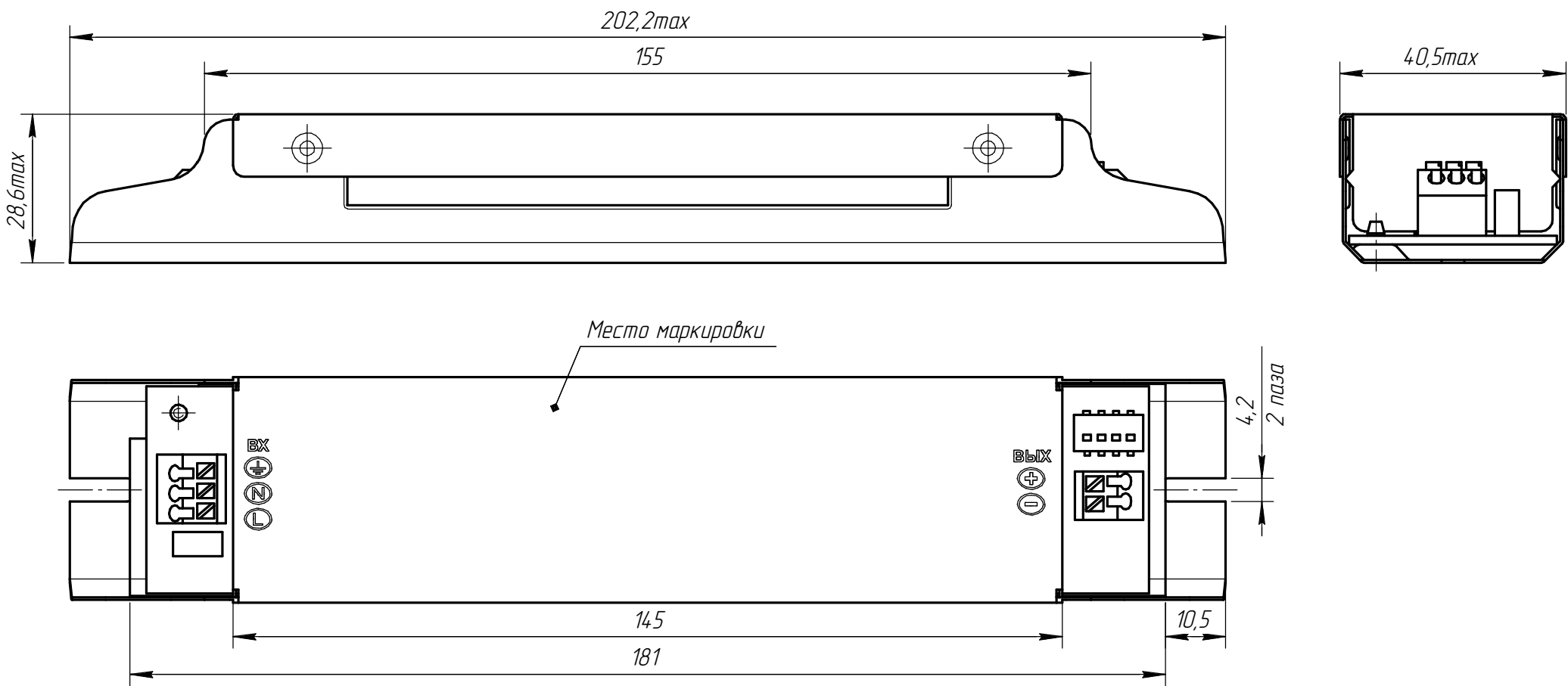
ИПС 40-50 Вт ТД 0100, 0105 (корпус А)
