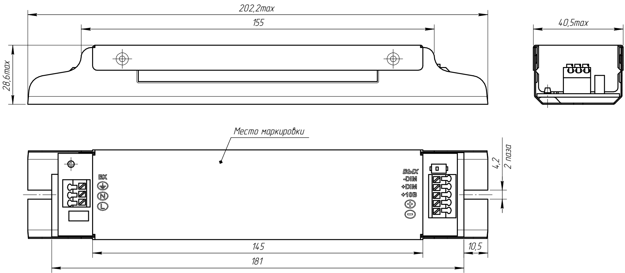
ИПС 50 Вт ТУ 0102 (корпус А)
